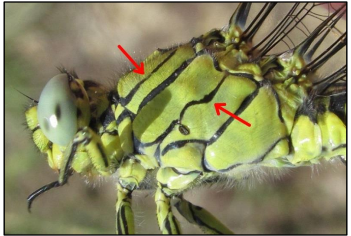
G. simillimus vs G. pulchellus des deux sexes
