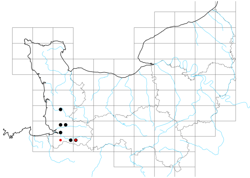
Distribution connue au printemps 2014 de Gomphus simillimus en Normandie (source : BDD du CERCION - 05/2014). Légende : points noirs = observations avant 2013, points rouges = en 2013, points rouges cerclés de noir = avant 2013 et en 2013.
