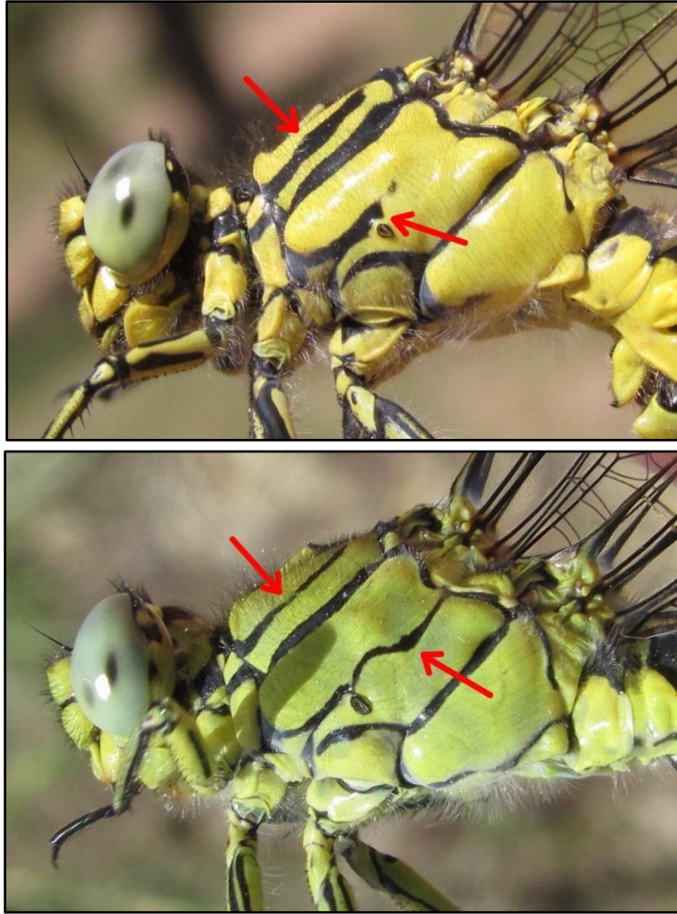
Figure 4 : Tête et thorax de G. simillimus en haut et de G. pulchellus en bas ; la flèche de gauche indiquant sur chacun la bande thoracique noire, large chez le 1 er /fine chez le 2 ème ; celle de droite la ligne mésopleurale interrompue chez le 1 er /complète-sinusoidale chez le 2 ème .
